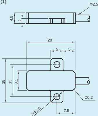
微型电感式传感器，Q8C微型扁方形外壳，DC 3线，供电电压：10...30 VDC
