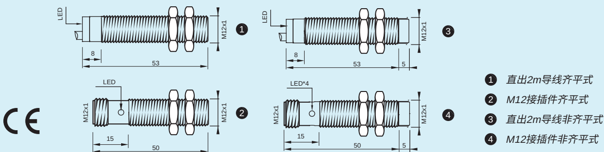
长距离圆柱形电感式传感器，M12 长距离型，DC 3线，供电电压：10...30 VDC
